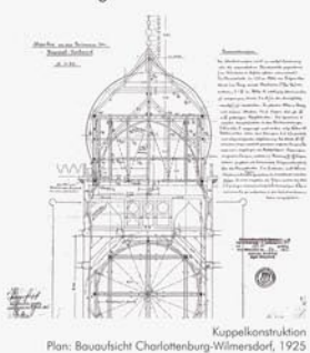
Plan: Bauaufsicht Charlottenburg-Wilmersdorf, 1925
